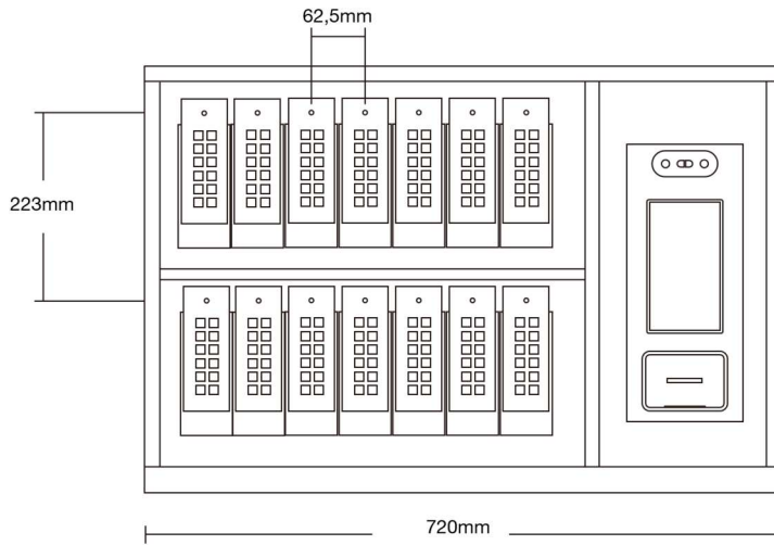
Vista Frontale
