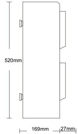
Vista Laterale
